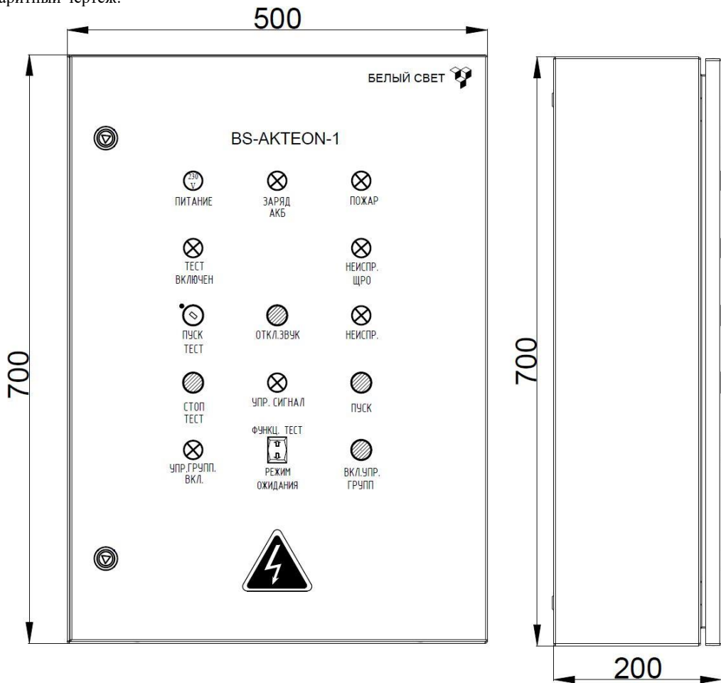
Рис. №2 Установочный чертёж.
