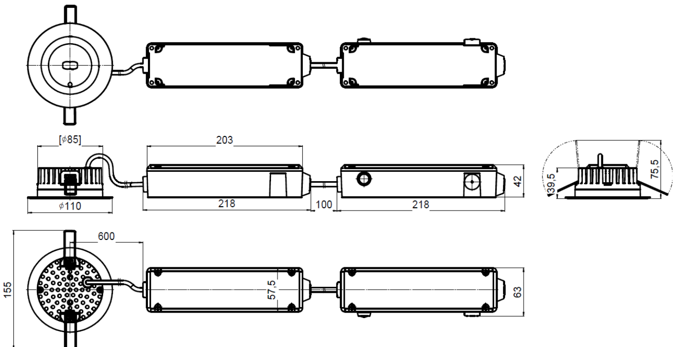
Рис. №2 Габаритный чертёж.
