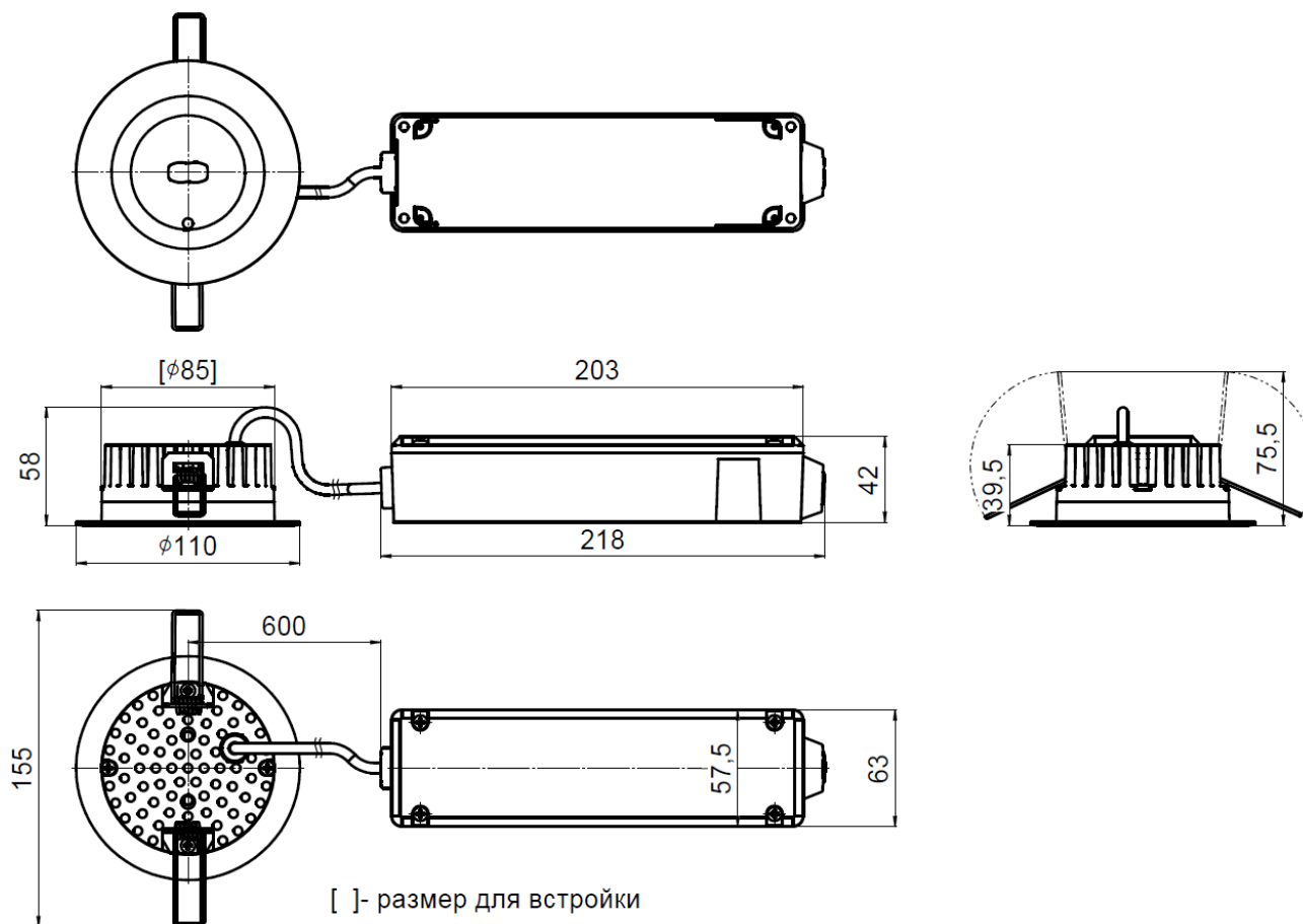
Рис. №2 Габаритный чертёж
