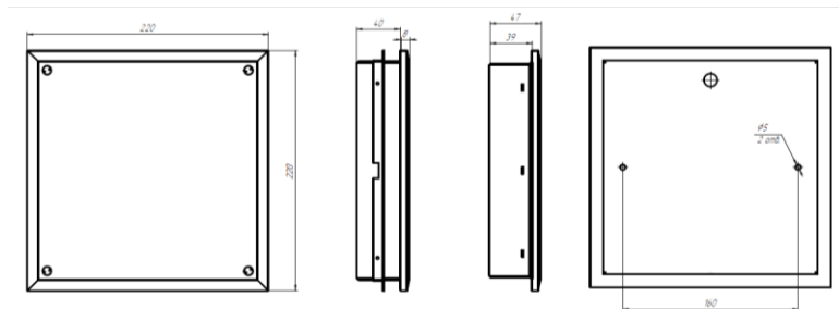
Рис. №2 Габаритный чертёж
