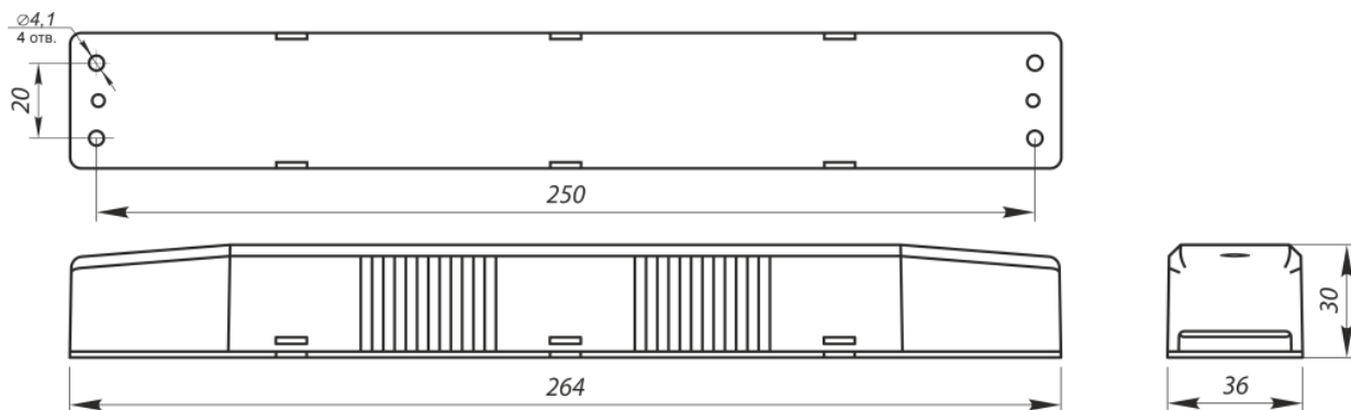
Рис. 8 Блок аварийного питания BS-STABILAR2- -LED
