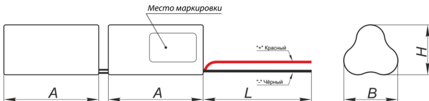
Рис.7 Габаритные размеры Батарея BS-3+3KRHT14/50-0.7/A-HB500-0-1 a27145
