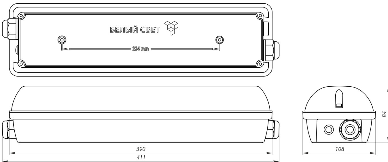
Рис. 8а Блок аварийного питания BS-STABILAR2-81-B1-LED BOX IP66
