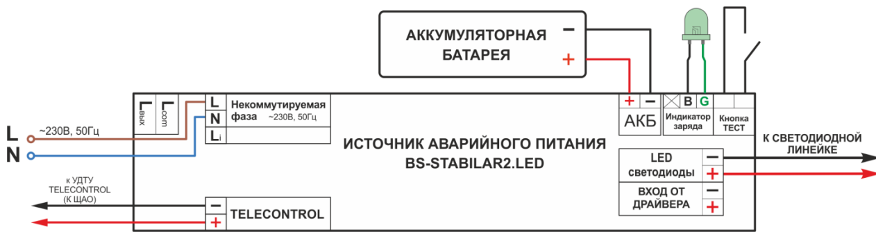
Рис. 2 Схема подключения BS-STABILAR2-81-B1-LED для аварийного светового прибора в непостоянном режиме:
