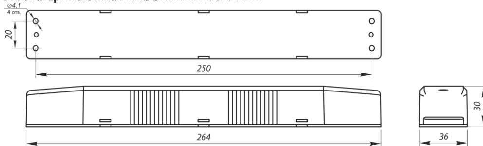
Рис. 8 Блок аварийного питания BS-STABILAR2-81-B1-LED
