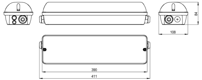
Рис. 10 Блок аварийного питания BS-STABILAR2-81-B1-UNI BOX IP65 (1,0-15 W / = 190-260 V)
