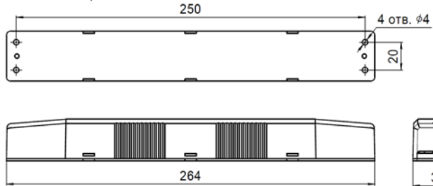
Рис. 7 Блок аварийного питания BS-STABILAR2-81-B1-UNI (1,0-15 W / = 190-260 V)
