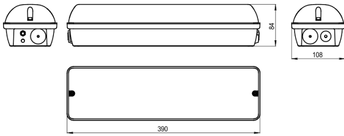
Рис. 9 Блок аварийного питания BS-STABILAR2-81-B1-UNI BOX IP30 (1,0-15 W / = 190-260 V)
