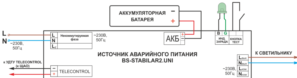
Рис. 2 Схема подключения BS-STABILAR2-81-B1-UNI (1,0-15 W / = 190-260 V) для аварийного светового прибора в непостоянном режиме:
