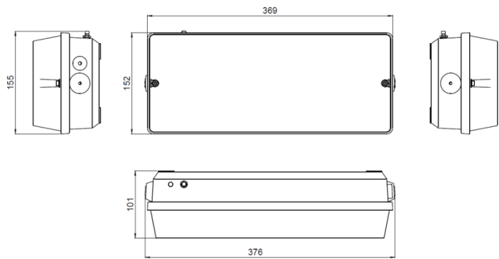
Рис. 9 Блок аварийного питания BS-STABILAR2-81-B2-UNI BOX IP30
