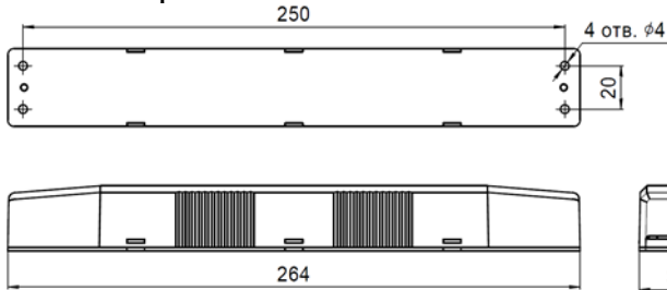
Рис. 7 Блок аварийного питания BS-STABILAR2-81-B2-UNI
