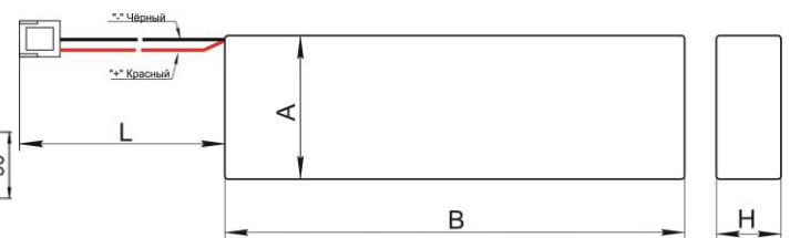
Рис.8 Батарея BS-10HRHT26/50-4,0/F-НВ500-VHR-3N-1
