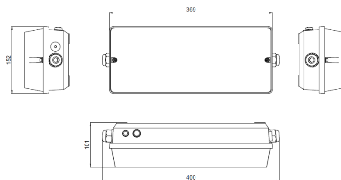
Рис.10 Блок аварийного питания BS-STABILAR2-81-B2-UNI BOX IP65
