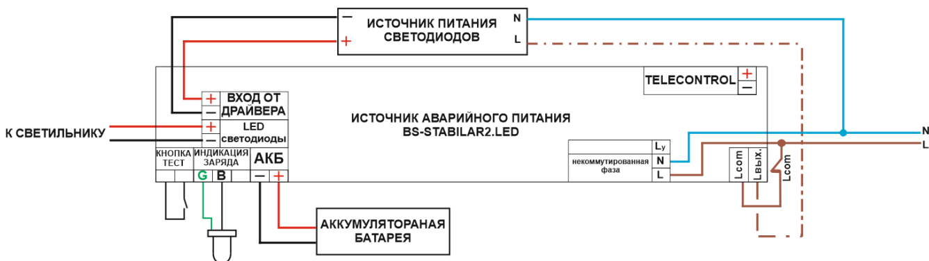
Рис. 2 Схема подключения BS-STABILAR2-81-B4-LED и BS-STABILAR2-83-B4-LED для аварийного светового прибора в непостоянном режиме:
