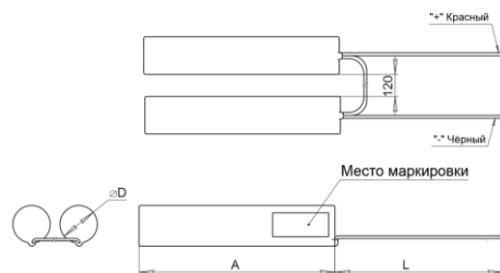
Рис.8 Батарея BS-3+3KRHT23/43-1.5/L-НВ500-0-1 а18268 Батарея BS-3+3KRHT33/62-4.5/L-НВ500-0-1 а18272
