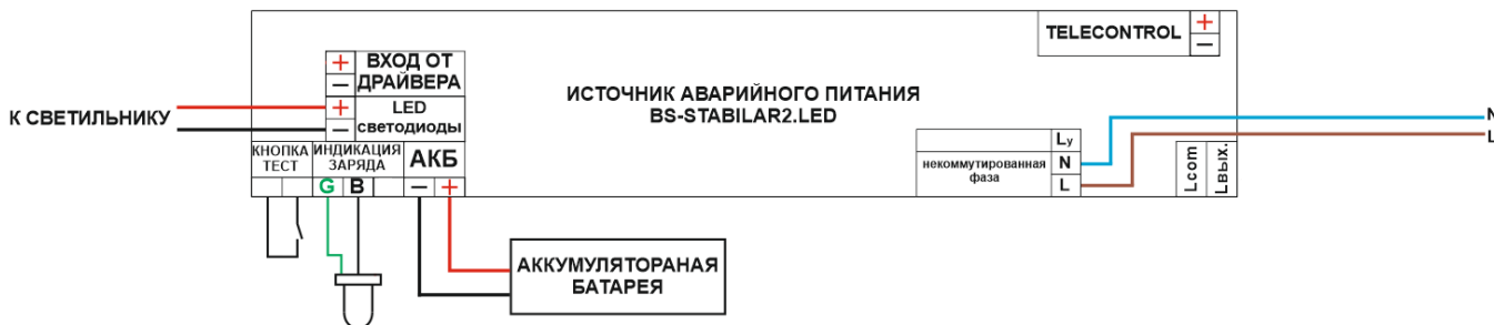
Рис. 2 Схема подключения BS-STABILAR2-81-B4-LED и BS-STABILAR2-83-B4-LED для аварийного светового прибора в непостоянном режиме:
