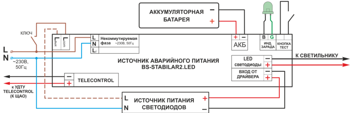
Рис. 1 Схема подключения BS-STABILAR-81-B3-LED и BS-STABILAR-83-B3-LED для аварийного светового прибора в универсальном режиме:
