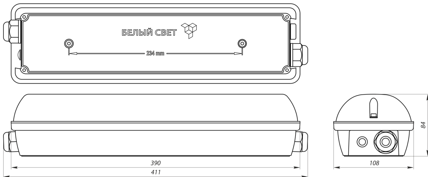
Рис. 8 Блок аварийного питания BS-STABILAR2-81/83-B3-LED BOX IP66
