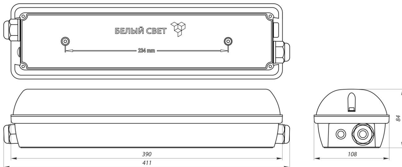
Рис. 8 Блок аварийного питания BS-STABILAR2-83-B2-LED BOX IP66
