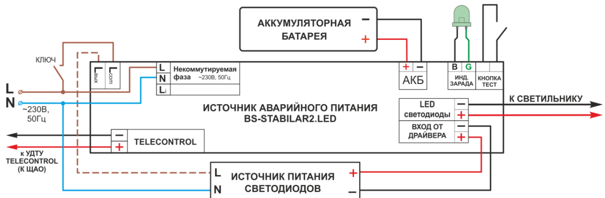
Рис. 2 Схема подключения BS-STABILAR2-83-B2-LED для аварийного светового прибора в непостоянном режиме:
