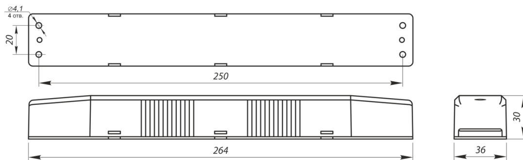
Рис. 8 Блок аварийного питания BS-STABILAR2-83-B2-LED BOX IP66
