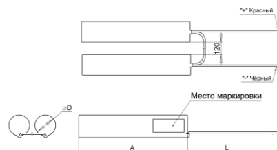
Рис.9 Габаритные размеры BS-3+3KRHT23/43-1.5/L-HB500-0-1 a18268
