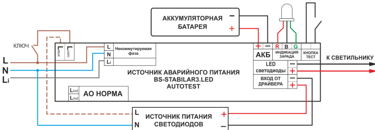
Рис. 2 Схема подключения BS-STABILAR3-81-B3-LED и BS-STABILAR3-83-B3-LED для аварийного светового прибора в непостоянном режиме:
