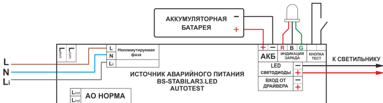
Рис. 2 Схема подключения BS-STABILAR3-81-B3-LED и BS-STABILAR3-83-B3-LED для аварийного светового прибора в непостоянном режиме:
