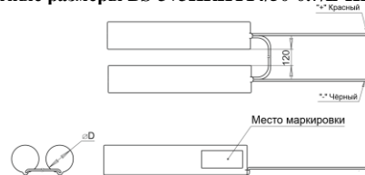
Рис.9 Габаритные размеры BS-3+3KRHT23/43-1.5/L-HB500-0-1 a18268
