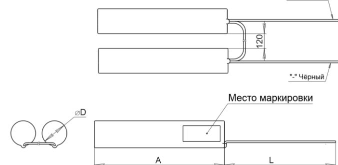
Рис.9 Габаритные размеры BS-3+3KRHT23/43-1.5/L-HB500-0-1 a18268
