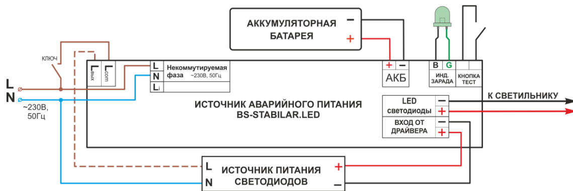
Рис. 1 Схема подключения BS-STABILAR-81-B2-LED и BS-STABILAR-83-B2-LED для аварийного светового прибора в универсальном режиме:
