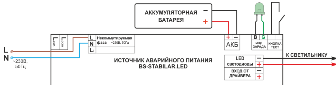
Рис. 2 Схема подключения BS-STABILAR-81-B2-LED и BS-STABILAR-83-B2-LED для аварийного светового прибора в непостоянном режиме:
