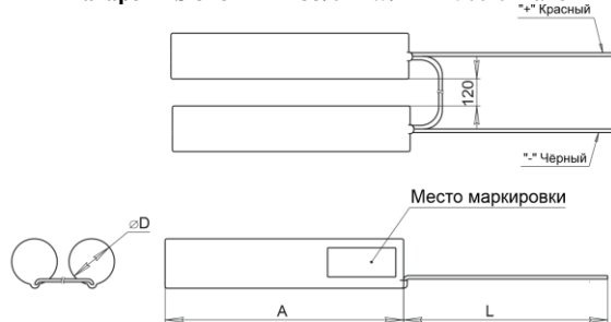
Рис.8 Батарея BS-3+3KRHT23/43-1.5/L-НВ500-0-1 а18268 Батарея BS-3+3KRHT33/62-4.5/L-НВ500-0-1 а18272
