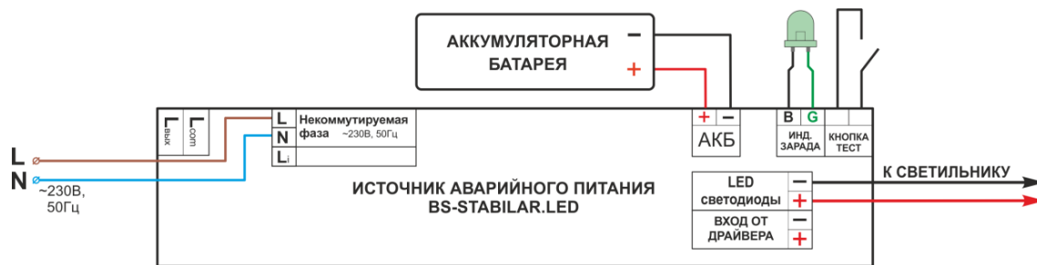
Рис. 2 Схема подключения BS-STABILAR-81-B3-LED и BS-STABILAR-83-B3-LED для аварийного светового прибора в непостоянном режиме:
