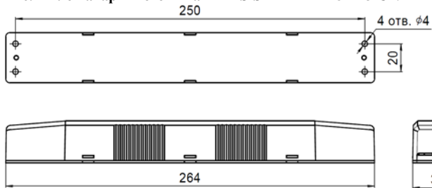
Рис. 7 Блок аварийного питания BS-STABILAR-81-B3-UNI
