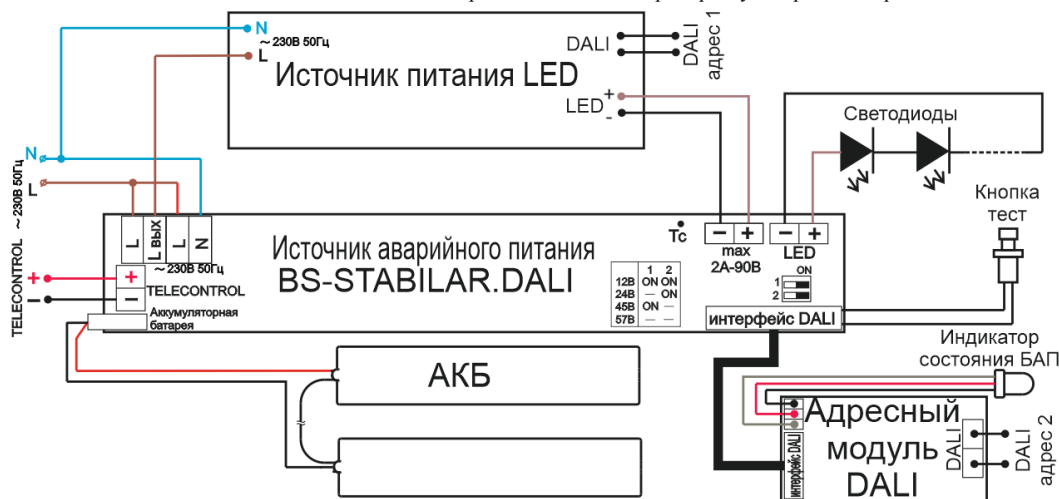
Рис. 1 Схема подключения BS-STABILAR-DALI для аварийного светового прибора в универсальном режиме:
