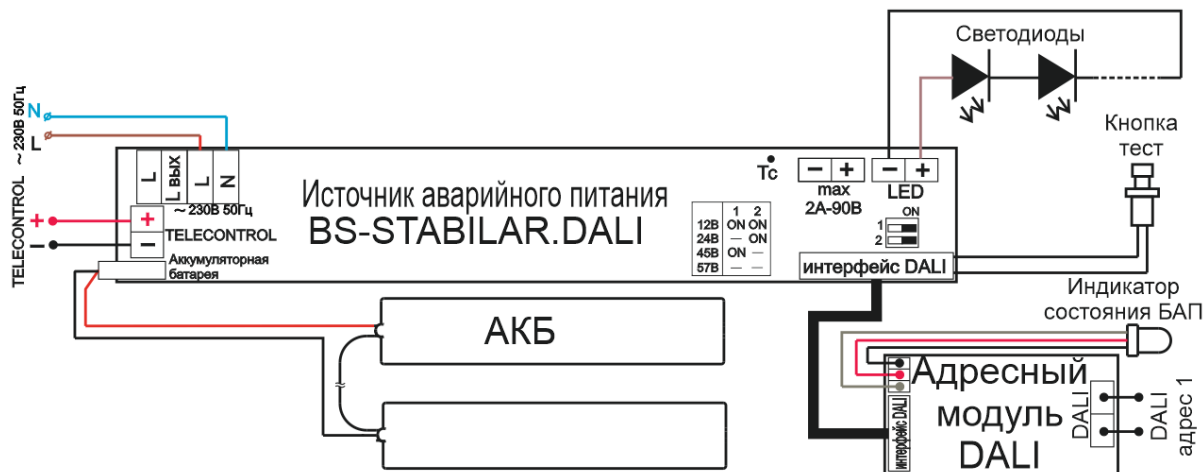
Рис. 2 Схема подключения BS-STABILAR-DALI для аварийного светового прибора в непостоянном режиме:
