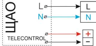
Рис. №1 Схемы подключения к групповой цепи питания и подключения к групповой цепи управления.
