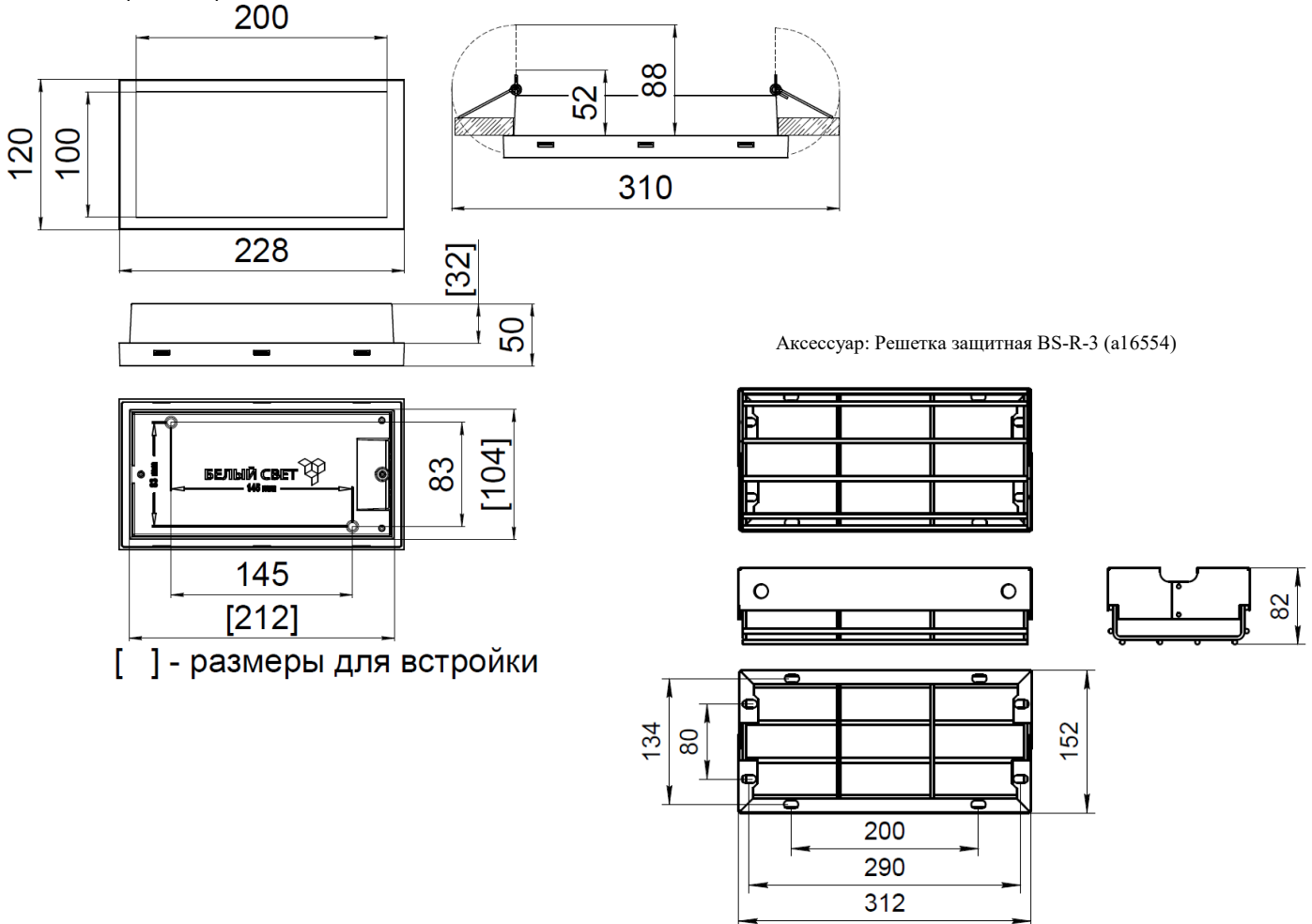
Рис. №3 Габаритный чертёж.
