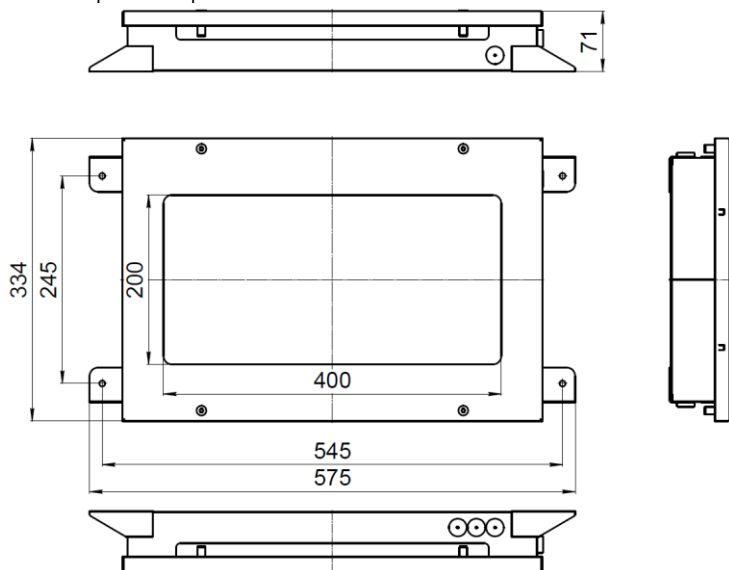
Рис. №5 Габаритный чертёж.
