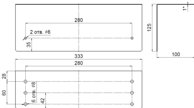
Рис. 4 – Аксессуар для крепления к потолку для BS-DBU-53-L2-INEXI3 Кронштейн BS-K-30 (a22635)
