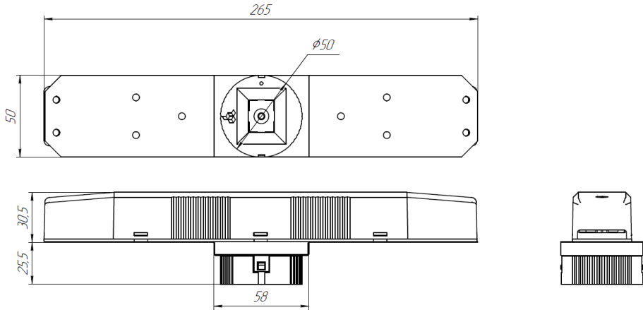
Рис. №2 Габаритный чертёж.
