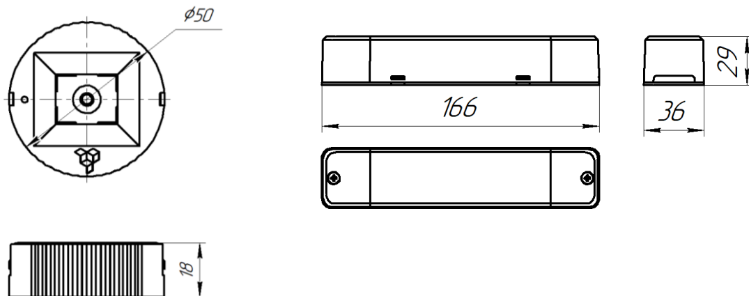
Рис. №3 Габаритный чертёж BS-ОКО-10-L1(2)-ELON GR и BS-ОКО-10-L1(2)-ELON GR BLACK.
