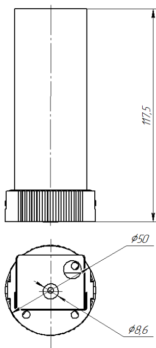
Рис. №2 Габаритный чертёж.
