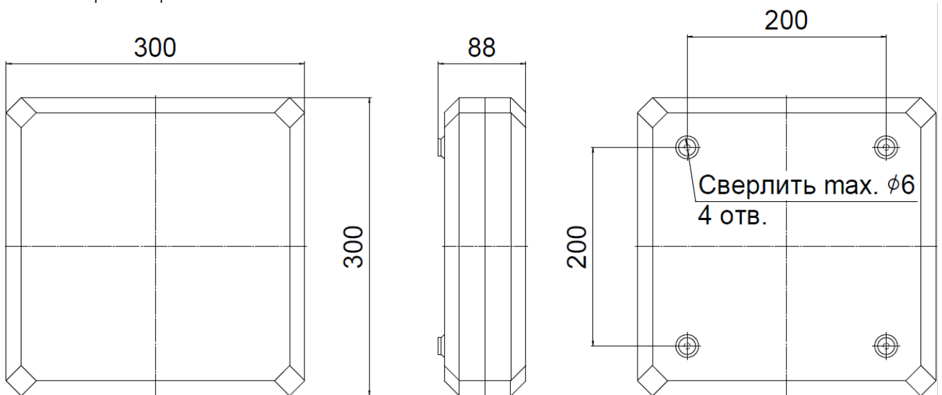
Рис. №2 Габаритный чертёж.
