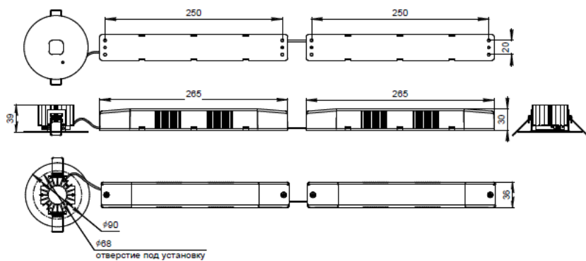
Аварийный светильник BS-RADAR-81-L4-STABILAR2
