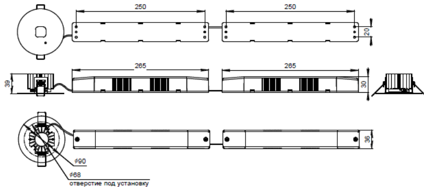
Аварийный светильник BS-RADAR-83- L1(L2; L3)-...
