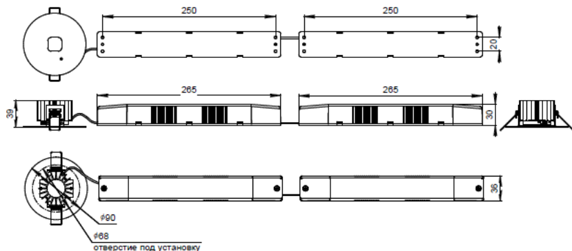
Аварийный светильник BS-RADAR-83-L4-STABILAR2
