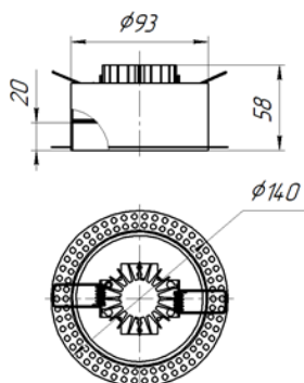
Стакан потолочный BS-SP-1
