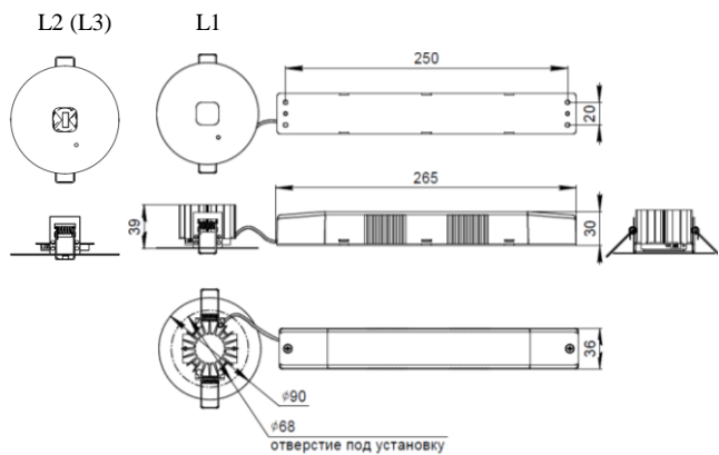
Аварийный светильник BS-RADAR-81-L1(L2; L3)-...
