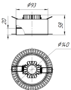
Рис. №4 Аксессуары Стакан потолочный BS-SP-1
