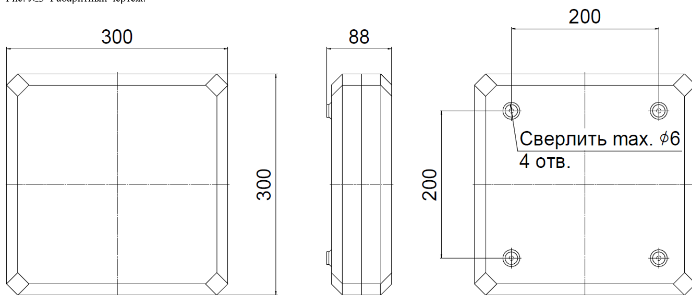
Рис. №3 Габаритный чертёж.
