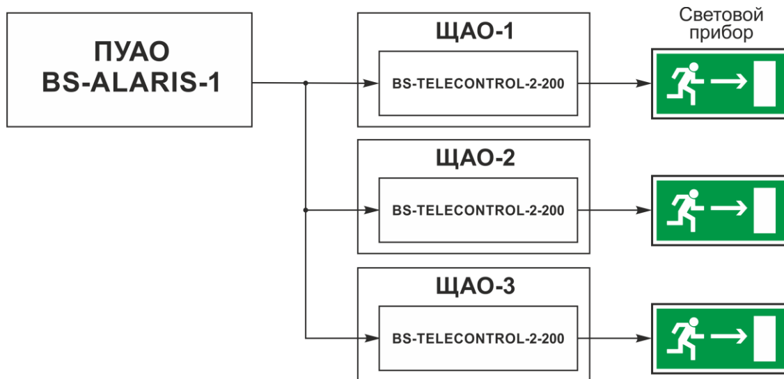
Рис 5. Схема подключения УДТУ BS-TELECONTROL-2-200 к ПУАО BS-ALARIS-1, для реализации Общего режима ожидания на объекте.
