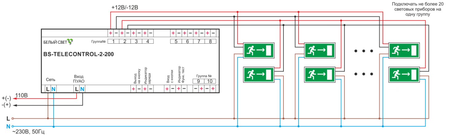
Рис. 3. Схема подключения УДТУ BS-TELECONTROL-2-200 к цепям питания и световым приборам групповых цепей управления.
