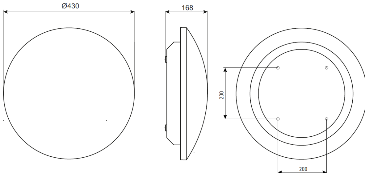
Рис. №5 Габаритный чертёж
