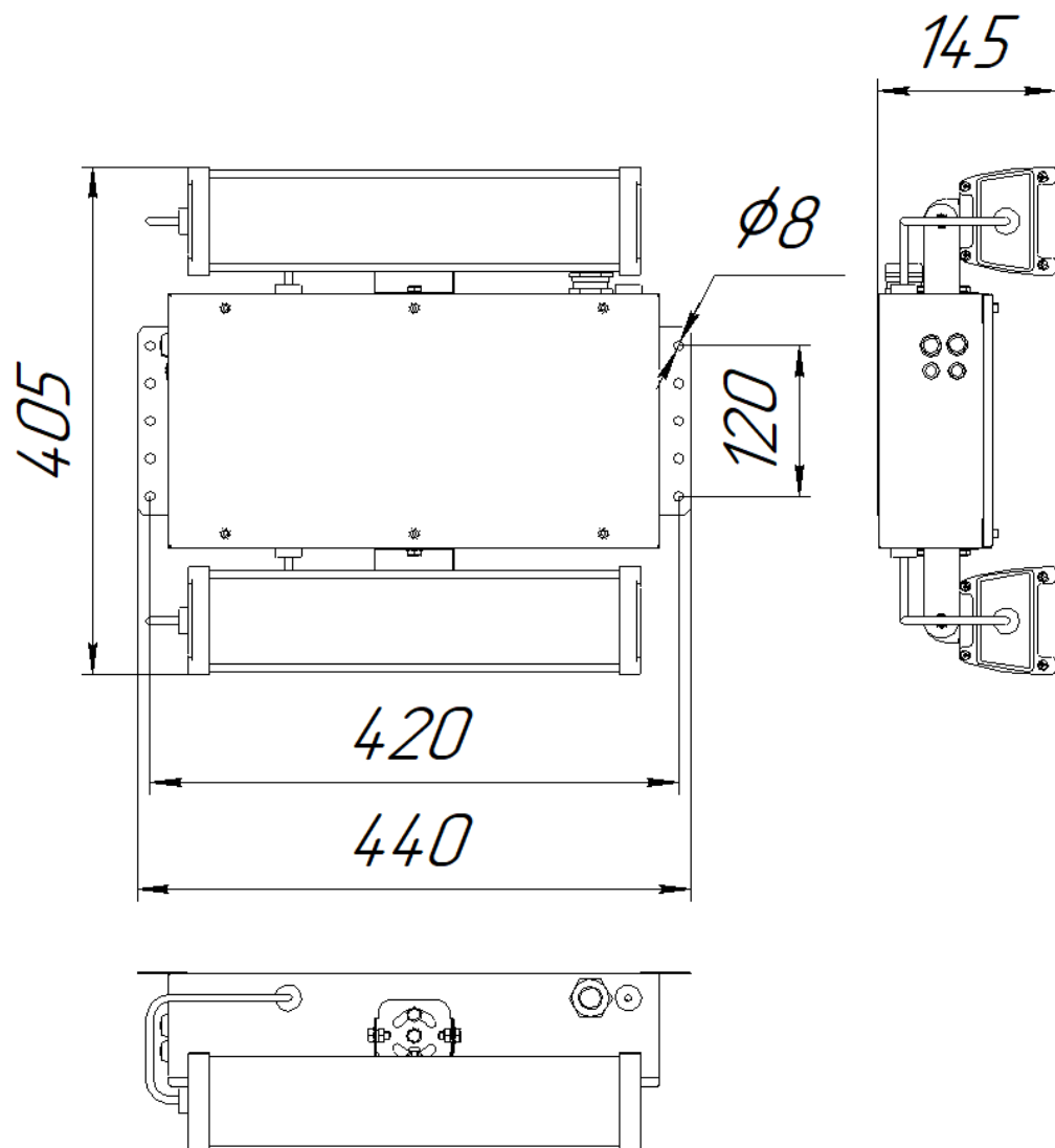
Рис. №2 Габаритный чертёж.
