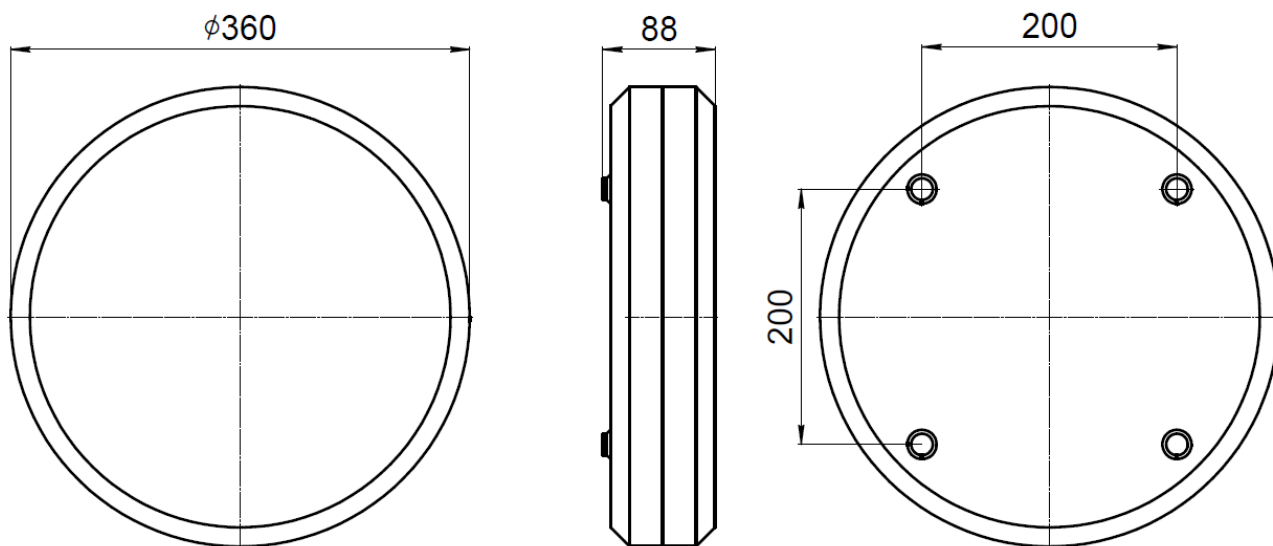
Рис. №5 Габаритный чертёж
