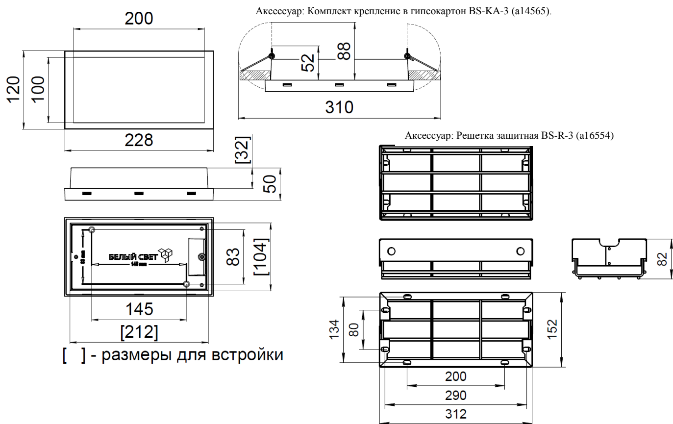
Рис. №2 Габаритный чертёж.
