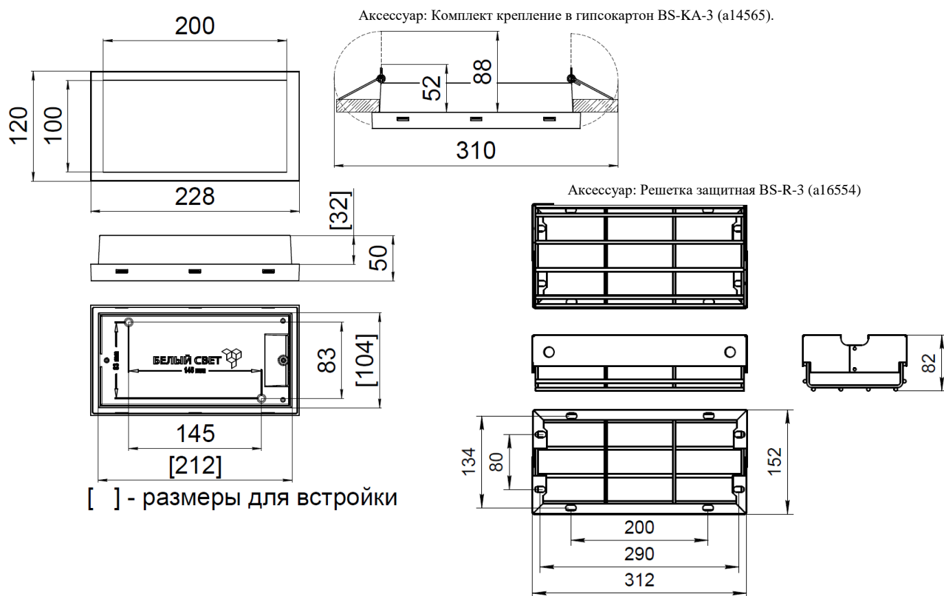
Рис. №2 Габаритный чертёж.
